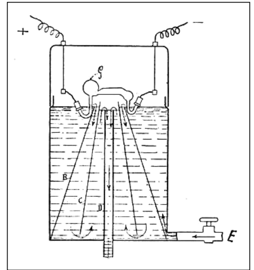
Principe van de Westinghouse-Cooper-Hewitt UV-sterilisator.
