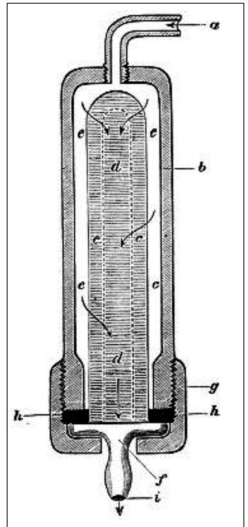
Doorsnede van een Pasteur - Chamberland - filter
