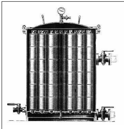
Batterij Delphin-filters voor gebruik in (semi-)permanente kantonneringen.
