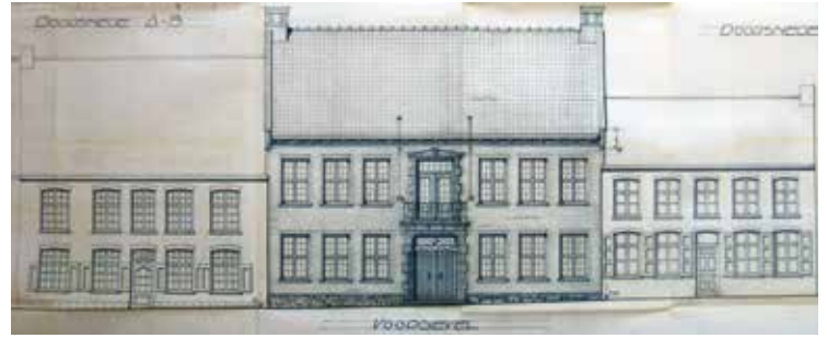
Gevelplan van de hand van architect Decreus uit Poperinge.
